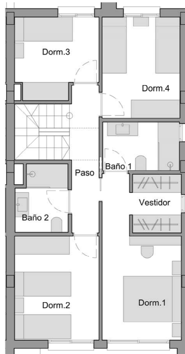
PLANTA PISO
