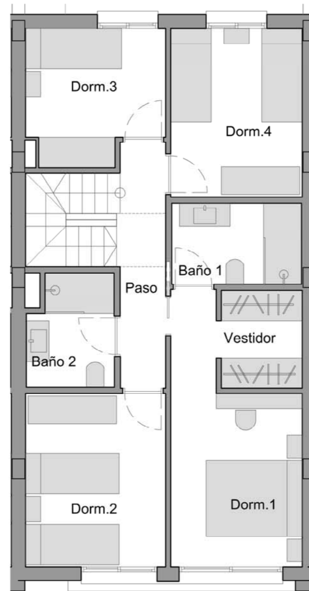
PLANTA PISO
