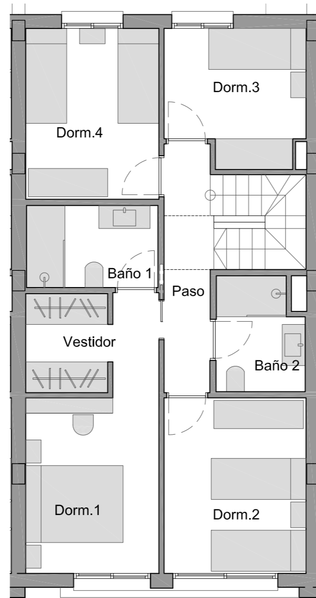
PLANTA PISO
