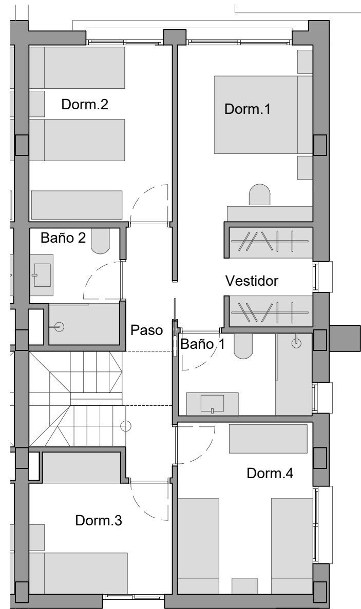
PLANTA PISO
