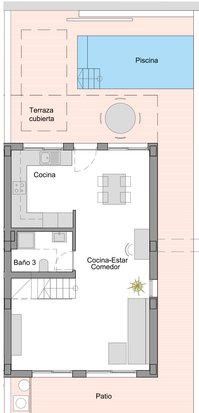
PLANTA BAJA
